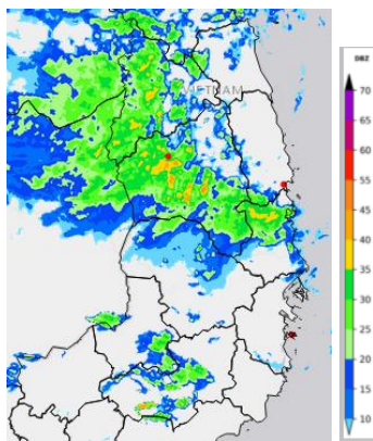
Ảnh radar thời tiết tại khu vực Tây Nguyên
